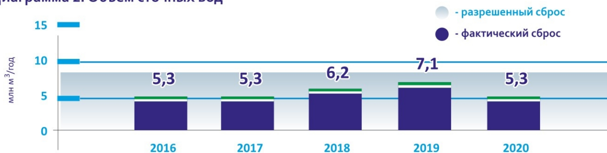
Диаграмма 2. Объем сточных вод
